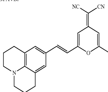
DPAVBi
