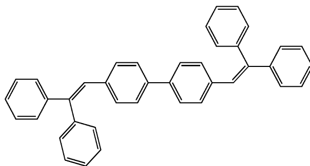
DPBVBi
